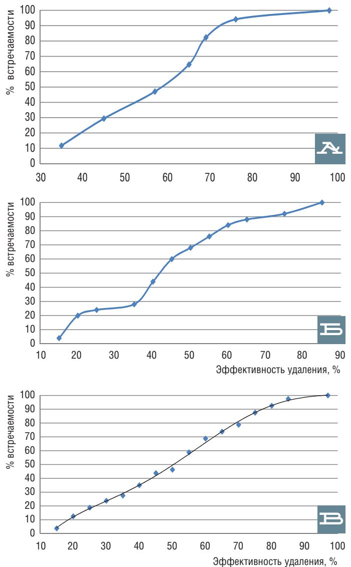
Рис. 3. РАСПРЕДЕЛЕНИЕ ПО ЭФФЕКТИВНОСТИ УДАЛЕНИЯ АЗОТА: а) для сооружений ОГСВ с ПП более 300 тыс. м 3 /сут.; б) для сооружений ОГСВ с ПП 100–300 тыс. м 3 /сут.; в) для сооружений ОГСВ с ПП менее 100 тыс. м 3 /сут.
